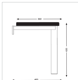
Banc avec support avant et fixation murale
