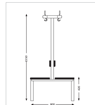
Banc double face avec barre à crochets et dossier
