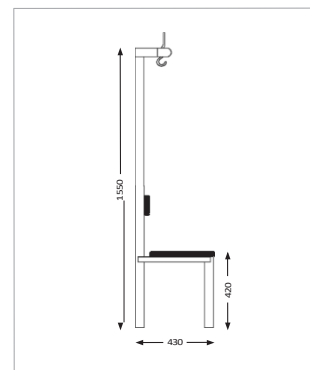
Banc simple face avec barre à crochets et dossier
