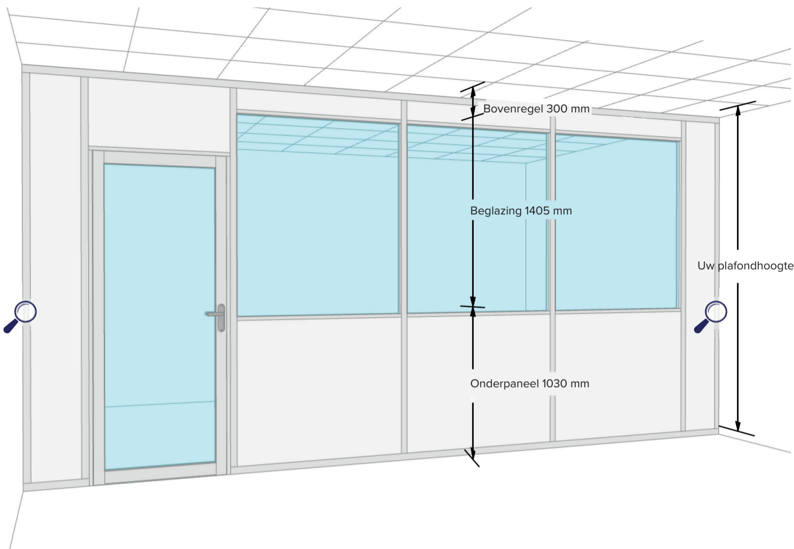
Bevestiging van de kantoorwand onder het plafond
