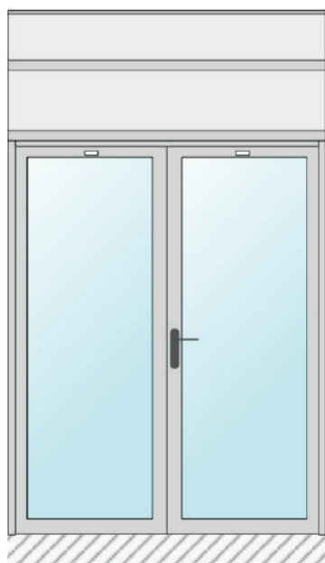
porte ALU double, Verre de sécurité (STADIP 33/2) Passage libre 1675 x 2100 mm
