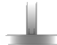
3 Raccordement de la façade à la cabine
