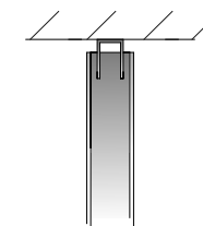
5 Raccordement mural avec un profilé en U comme joint creux
